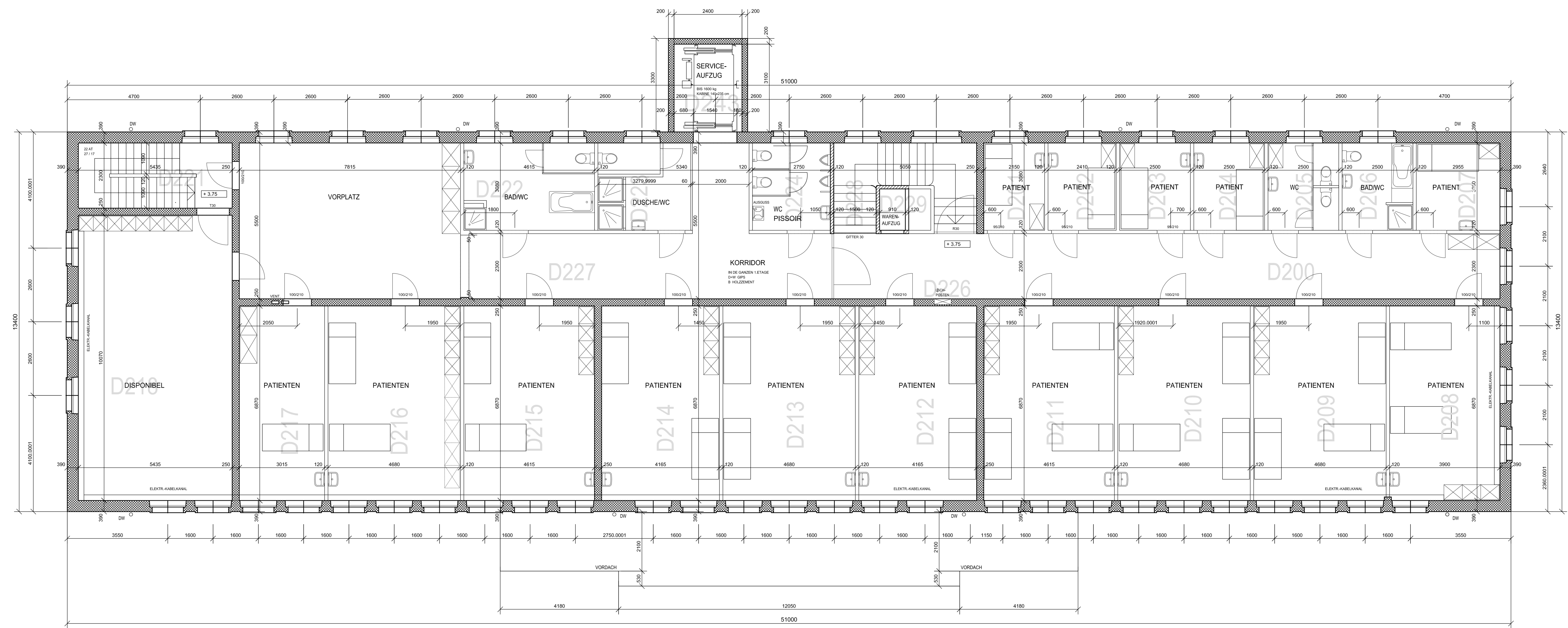
GRUNDRISS 100
